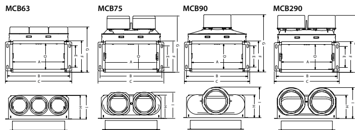
DE Wandanschlussgehäuse - Anschlüsse oben
